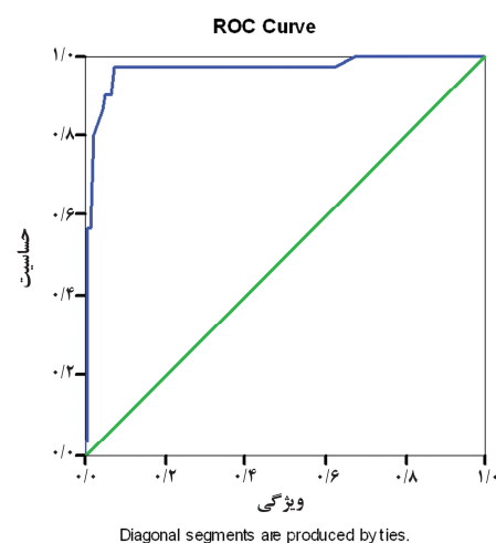
نمودار ۲: میزان accuracy سطح زیر منحنی
