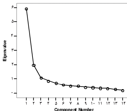
نمودار ۱: نمودار ارزش‌های ویژه و الگوی وزن‌های عاملی پرسش‌نامه‌ی CIUS
